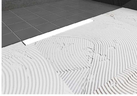
PH PRODRAIN Duş kanalı zemin izolasyonu / Apply waterproofing
